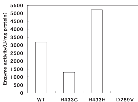
図3 酵素活性
