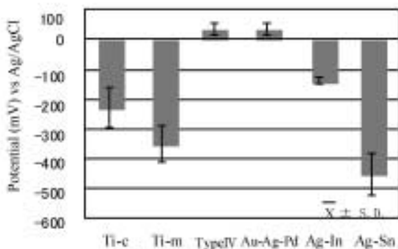
図13 各金属材料の自然電位
