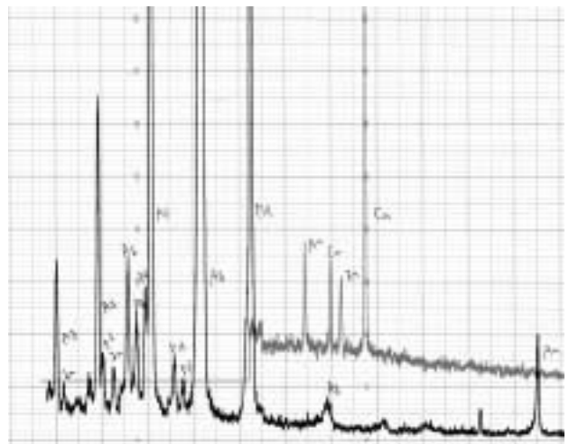
図4 EPMA分析結果 検出された特性X線の波形。図のチャートでは金, パラジウム, 銀, 銅, インジウム, 亜鉛が検出された。
