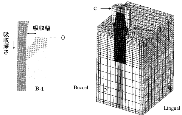
図1 左図はカップ状吸収形態のシェーマ。それぞれの方向に表1で示す値だけ吸収するものと仮定した。右図はBaseモデルでの三次元有限要素解析モデル (Cross sectional view)。それぞれ、a (皮質骨)、b (海綿骨)、c (インプラント体および上部構造) とした。
