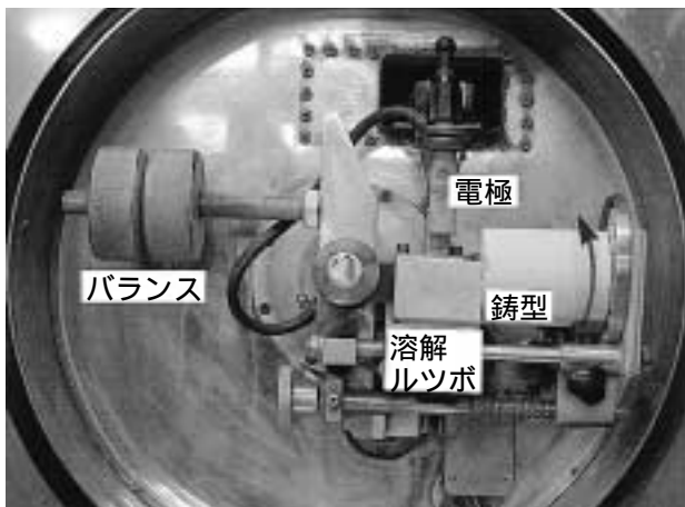
図10 チタンウマー-VF中心部写真
