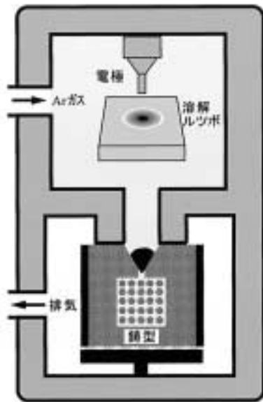
図1 サイクラーク模式図：溶湯落下の瞬間
