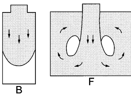
図15 鑄型内の流れの代表パターン
