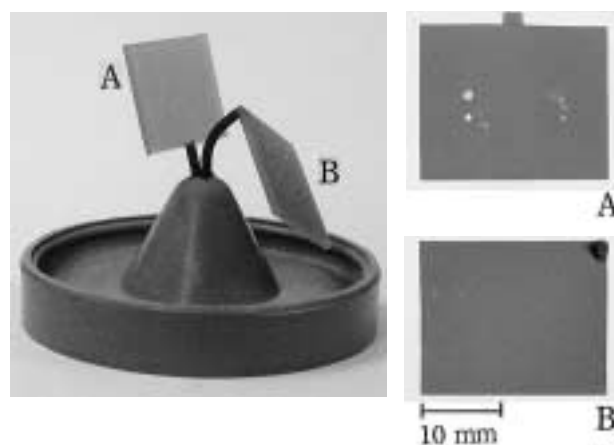
図16 スプルー植立写真と鑄造体透過X線写真
