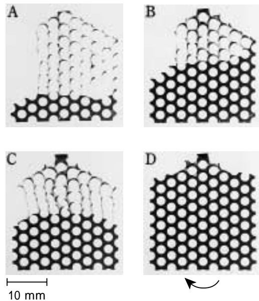
図8 鑄造体X線透過写真：A、B、C、Dは図7の対応する部位にスプルー植立、矢印は回転方向、AとBはコリオリの力による違い、CとDは専用グラファイト湯口形状の影響
