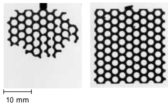
図3 鑄造体X線透過写真：左は通常法，右はコーンタイプ遮蔽箔使用
