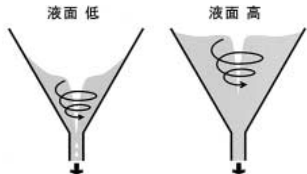
図13 鑄型クルシブルで発生する吸い込み渦模式図
