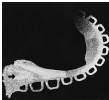
図11 単純化した金属床鑄造体：流れ模様観察のためパラジウムで標識
